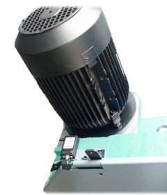
Motor med elektronisk variator: bandrotation från 18 till 90 m/minut
