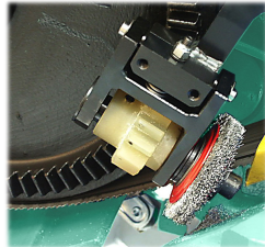
Mekaniskt drivet spårrenshjul som rengör bandet från spånor
