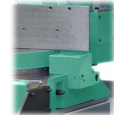
Justerbart bakre anhåll för öppning av skruvstycket max 450 mm
