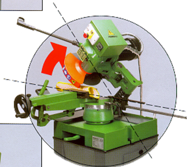
Kapning 45° vertikalt
